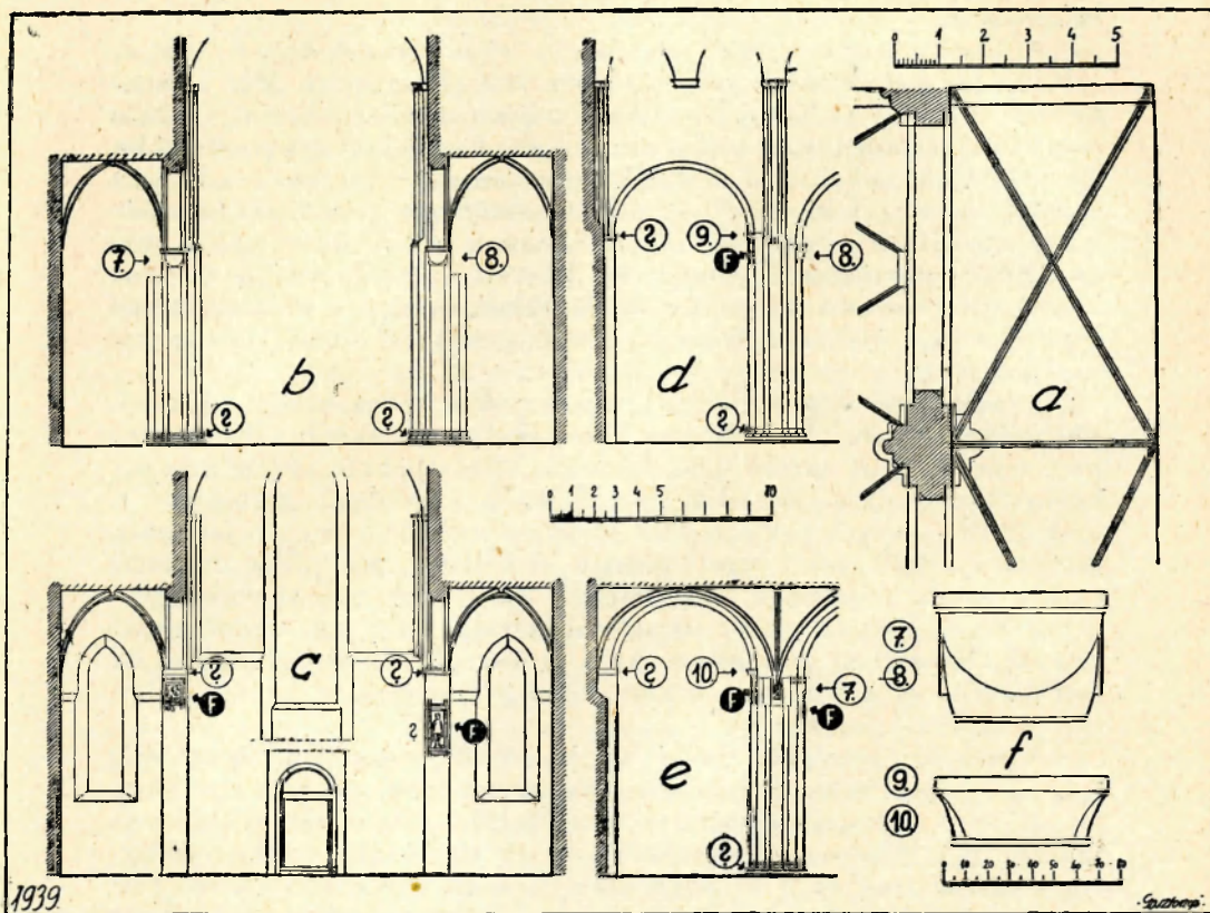
Énekkarzat részletei Schmidt felvételi rajzai szerint. a) északi mellékhajó és énekkarzati pillérek alaprajza, b) énekkarzati pillérek nézete, c) nyugati homlokfal belső nézete, d) északi főhajófal nézete a főhajóból, e) déli főhajófal nézete a mellékhajóból, F) freskómaradványok helye, 7—8—9—10. f) pillérfejezetek.
