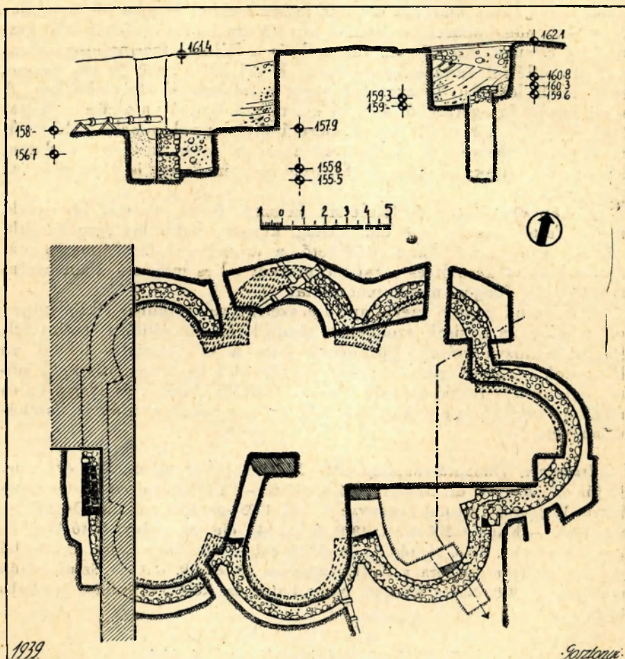
Hétkaréjos épület (L.) felvételi rajza.
