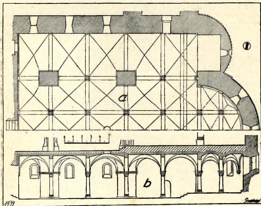
Altemplom alaprajza és metszete Schmidt felvételi rajza szerint.
