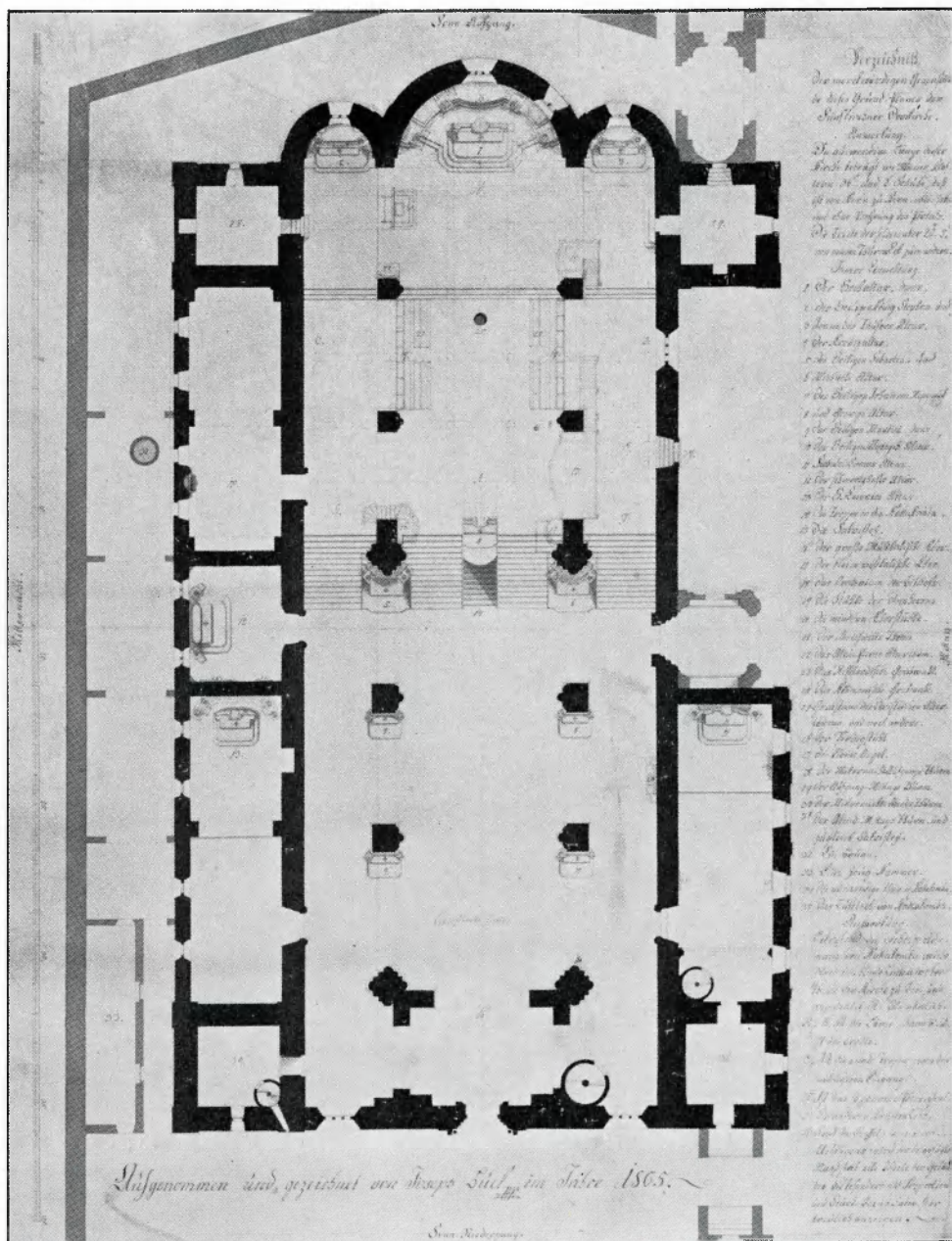
A pécsi Szent Péter székesegyház 1805. előtt. Buch József felvétele és rajza. (Székesegyházi Múzeum.) V. ö. 12. sz. rajz, 195. o.
