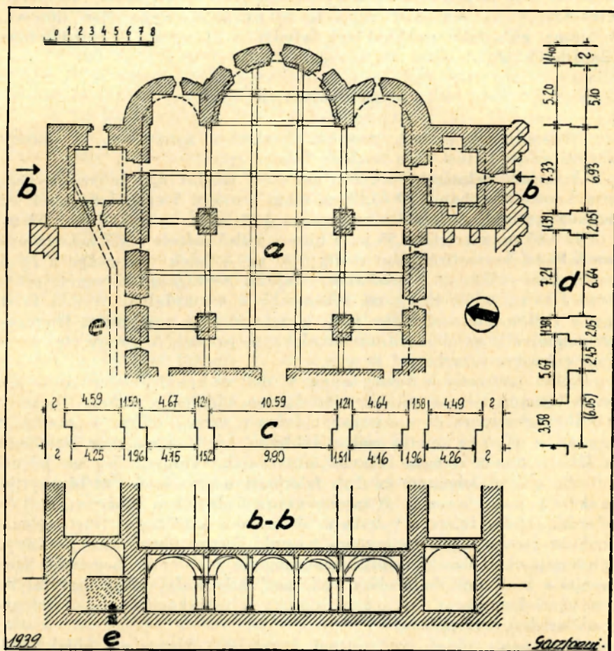
A keleti toronypár és altemplom helyzete a Schmidt-féle átépítés előtt Buck és Schmidt felvételi rajzai alapján. c-d méreetszelvény.
