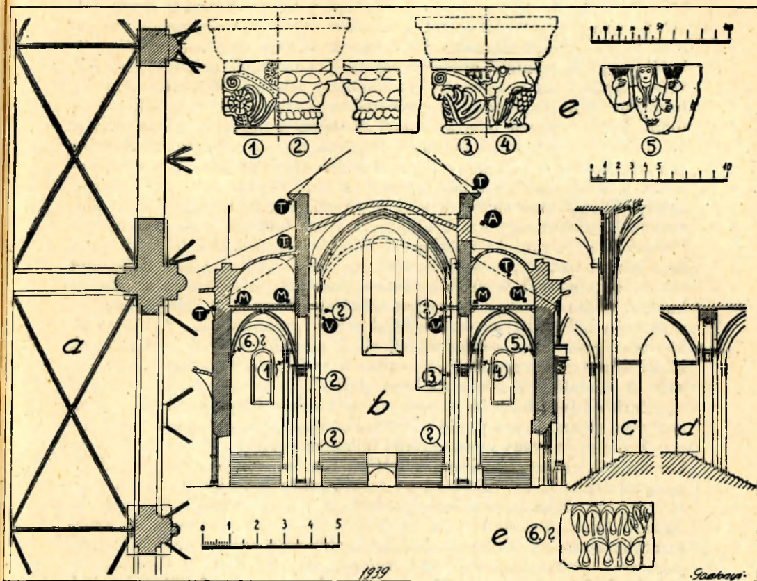
Szentély diadalívének részletei Schmidt felvételi rajza szerint. a) északi oldal-hajó és pillérsor alaprajza, b) diadalív nézete nyugatról, c) főhajó felől, d) mellék-hajó felől. A főhajóablakok helye, M. mennyezet, T. tető, V. diadalív válla. 1, 2, 3, 4, 5, 6. (e) pillérfejezetek és konzolok.
