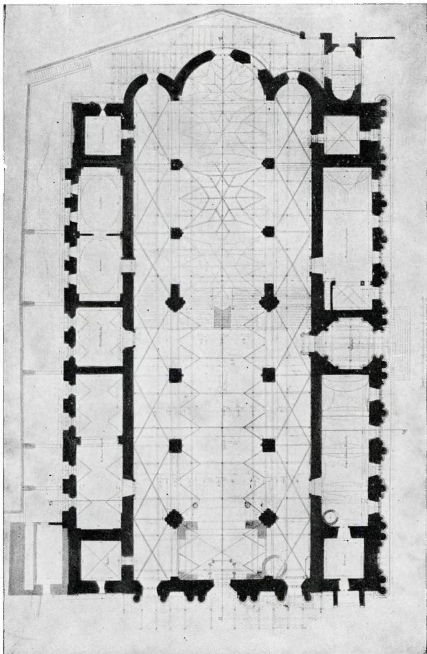
A pécsi Szent Péter székesegyház 1882. előtt. Schmidt Frigyes felvétele és rajza. (Székesegyházi Múzeum.) V. ö. 12. sz. rajz, 193. o.
