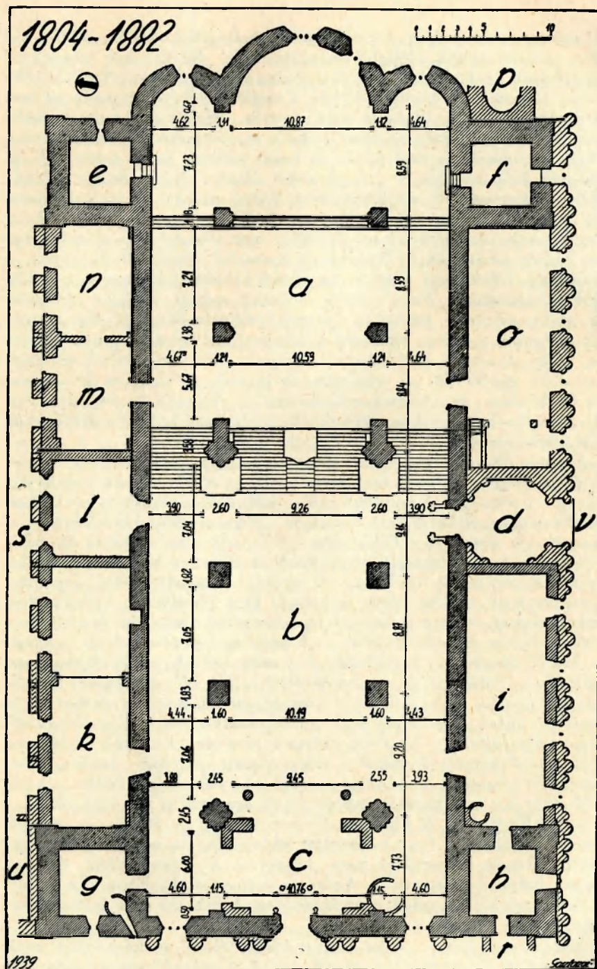
A székesegyház alaprajzi állapota a Pollák-féle átépítés előtt és változása a Schmidt-féle restaurálásig. a szentély és altemplom, b néphajó, c énekkarzat, d bejárati csarnok, e–h tornyok, i–l és o kápolnák, m–n sekrestye, p–s átjárók, u kamra, v déli főbejárat.
