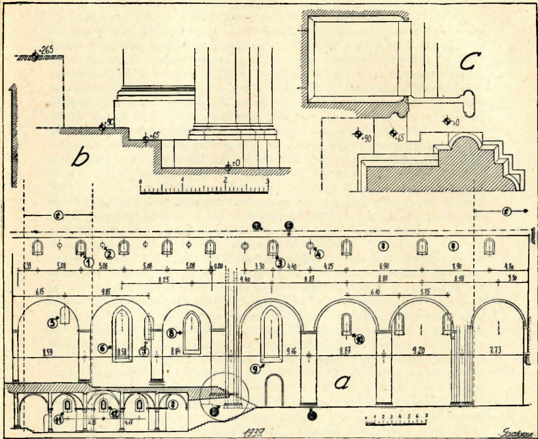
Hajóválasztó pillérrendszer és hajóablakok Schmidt felvételi rajzai szerint. a) déli fő és mellékhajófal a főhajóból nézve, b) déli diadalt pillér nézete és c) alaprajza, F. románkori famennyezet vonala, P. románkori padlósík, T. románkori párkánymagasság. 1—12. ablakok.
